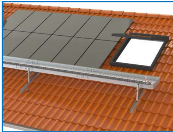
C-Gleiter 500
