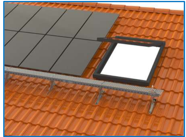
C-Gleiter 250
