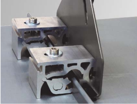
Laufroststützen auf Doppelstehfalz:
