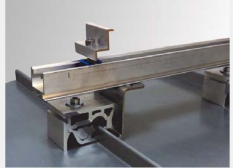
Solarhalter auf Doppelstehfalz:
