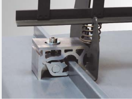
Schneefangstützen auf Winkelstehfalz:
