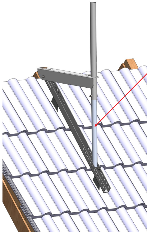
Trägerprofil
