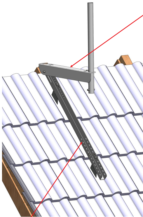
Trägerprofil
