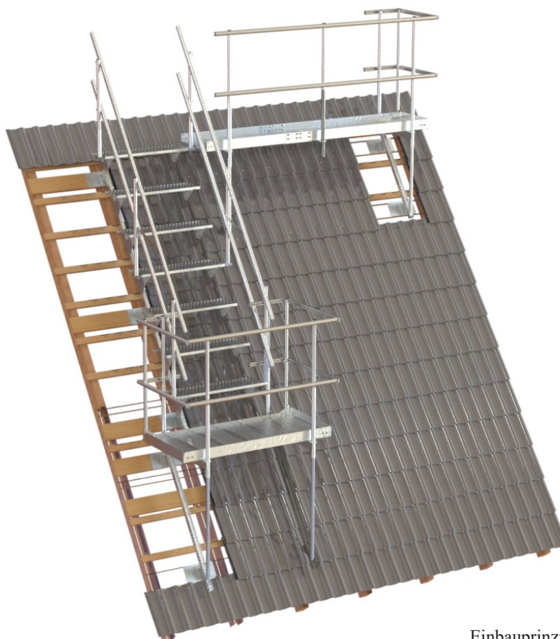
Einbauprinzip
