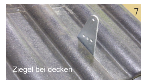
Deckelement + ca. 1cm im Bereich des Schwer-tes aussparen / schlitzen (Rasterunabhängig)
