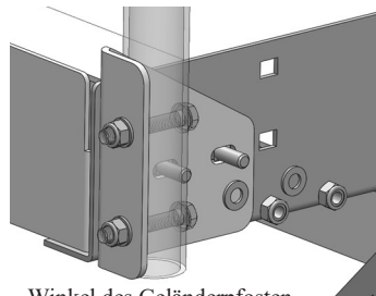
Winkel des Geländerpfosten
