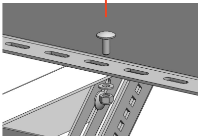
[Schraubensatz E]
