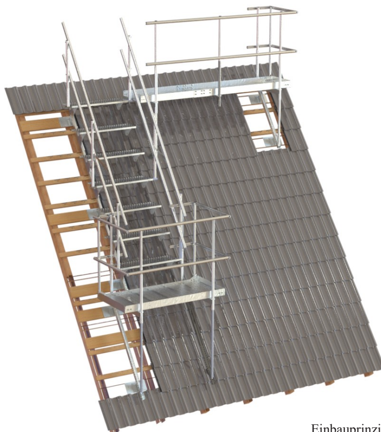
Einbauprinzip
