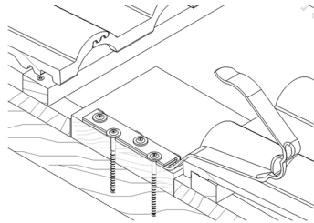
Schema 4 Typ B geschraubt
