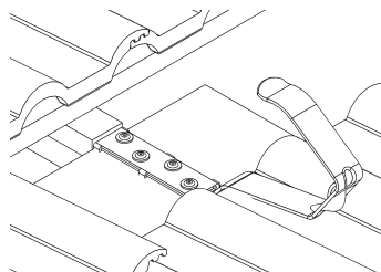
Öse Sicherungsschuh Richtung Hakengrund
