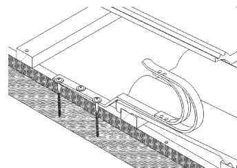
Schema 5 Typ A genagelt; Typ B geschraubt
